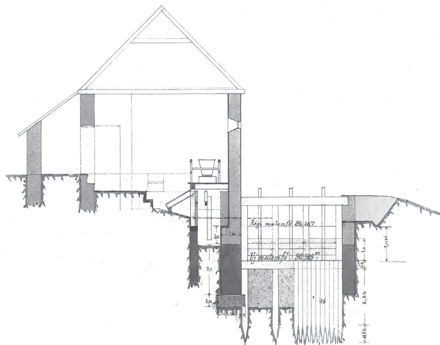
Zsilip hosszmetzete.
