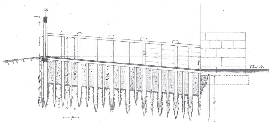
Zsilip hosszmetzete.
